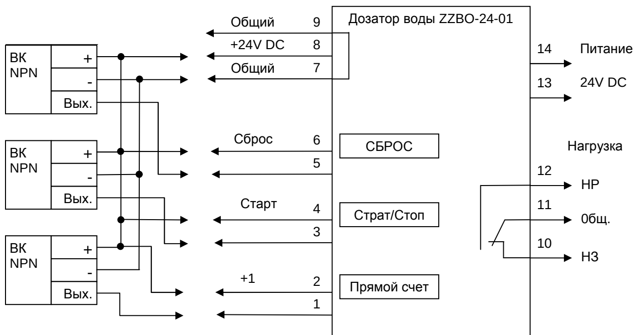
Подключение к дозатору NPN выключателей
